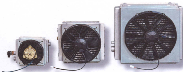
Série refroidisseurs d'huile/équipés ou non de moto-ventilateur/aluminium Serie of oil coolers / With or without fan/ aluminium
