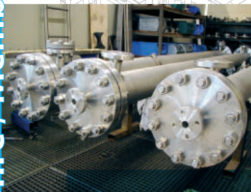
Druckrohre in Sideportausführung PN 100, das Hauptrohr ist aus pass- genauem Rohr für die Membran- technik Pressure vessels of side port type at pressure stage PN 100, the main pipe is specially made for the membrane technique
