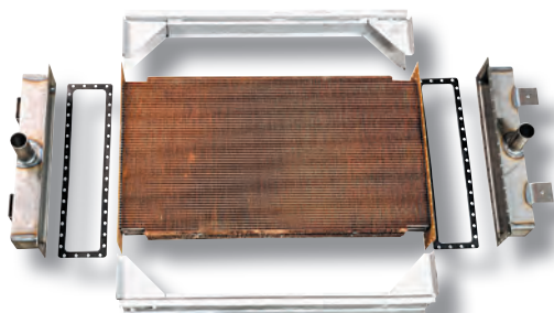
Radiateur non assemblé - Conception cuivre/acier
