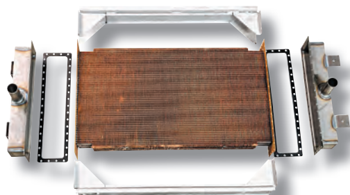
Radiateur non assemblé - Conception cuivre/acier
