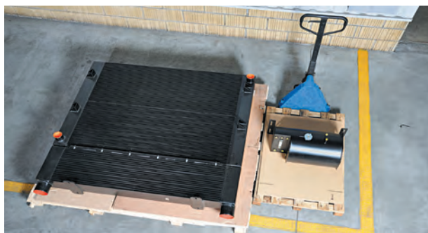
Combiné eau/air aluminium dim. hors tout en mm 1800x1200x250 + vase d'expansion
