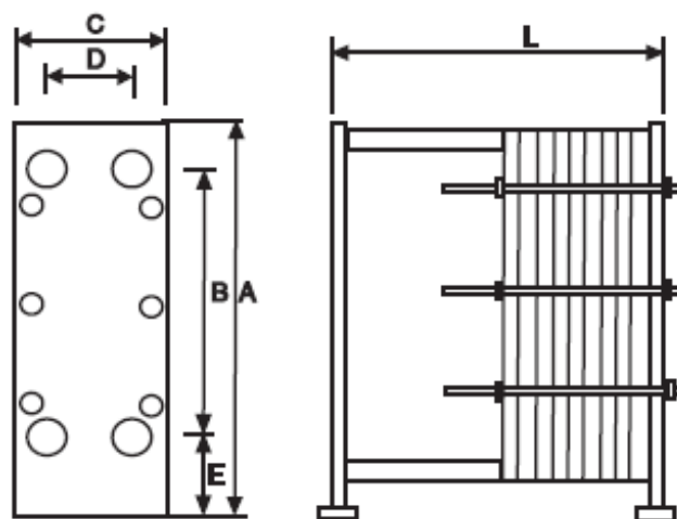
Параметры пластинчатых теплообменников Машимпэкс (GEA) VT80:
