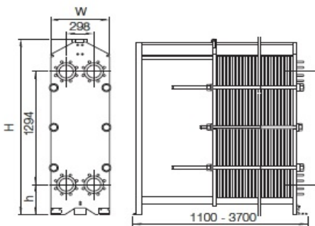
Габаритный чертеж, Размеры в мм
