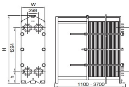
Габаритный чертеж, Размеры в мм
